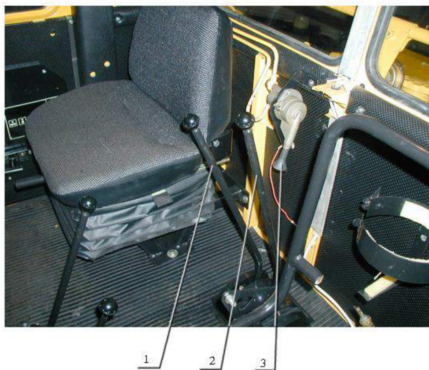
Рис. 10. Оборудование кабины
