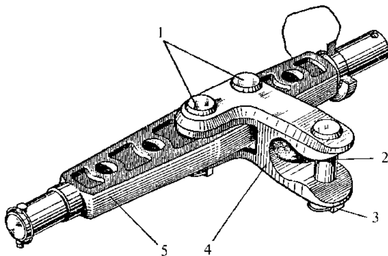
Рис. 60. Скоба прицепная
