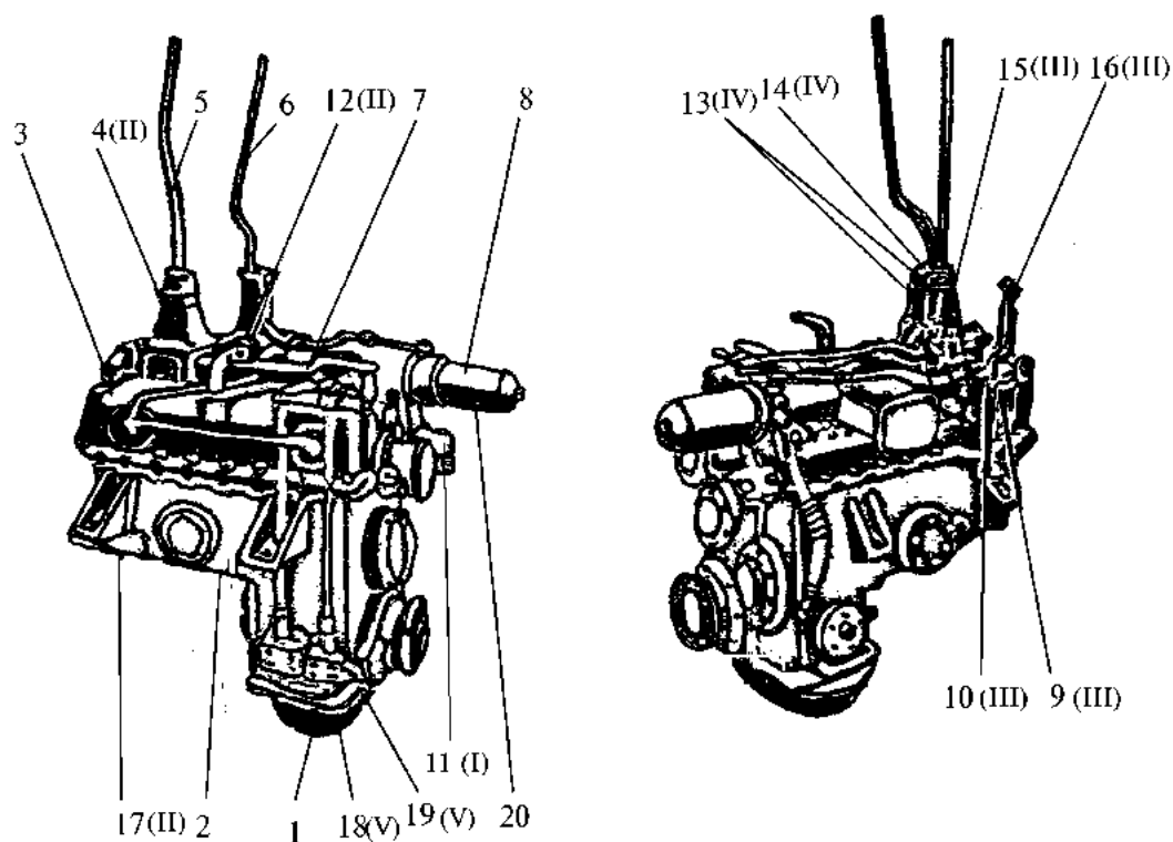
Рис. 26. Коробка передач
