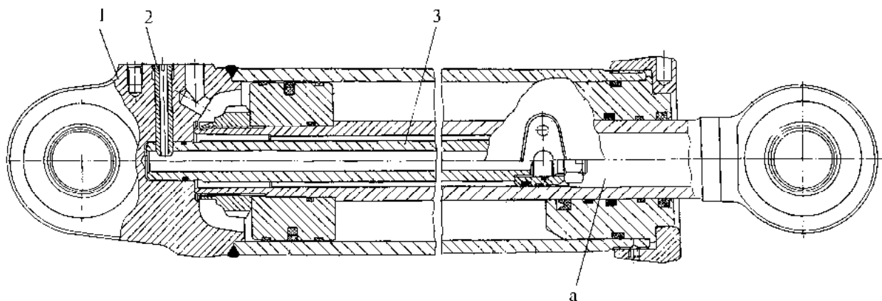
Рис. 56. Гидроцилиндр поворота для гидросистемы с гидрораспределителями ГА-35/ГА-36 1 - крышка задняя; 2 - стопор; 3 - шток следящий
